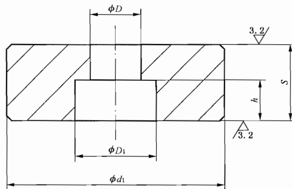
图 1 垫圈
