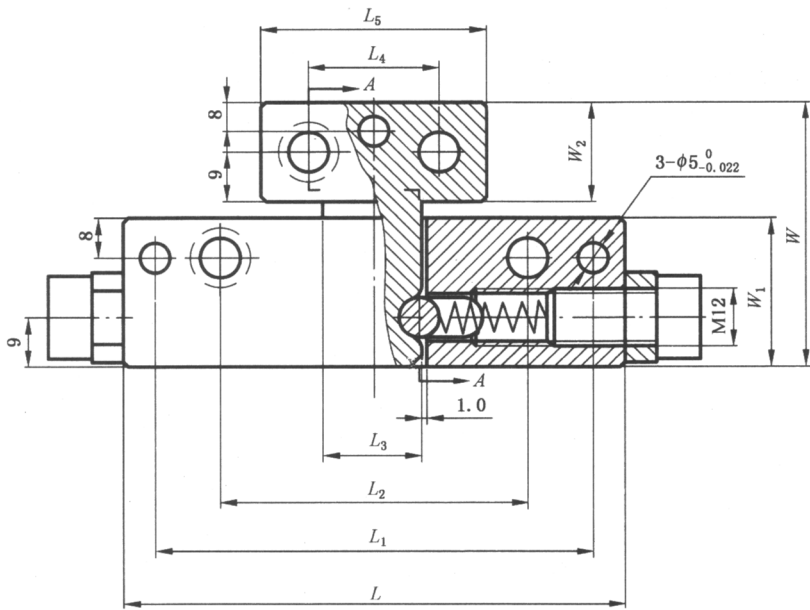
图 1 矩形拉模扣
