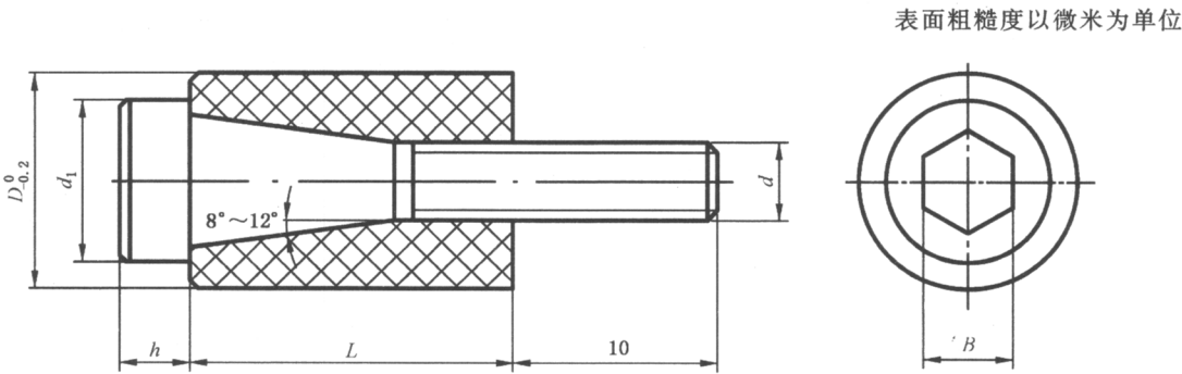
图1 圆形拉模扣
